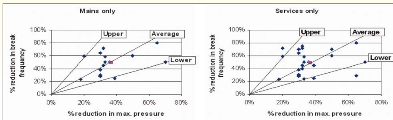
FIGURA 2: INFLUENZA DELLA GESTIONE DELLA PRESSIONE SULLA FREQUENZA DELLE ROTTURE DI RETE (MAINS ONLY) E PRESE (SERVICES ONLY)
