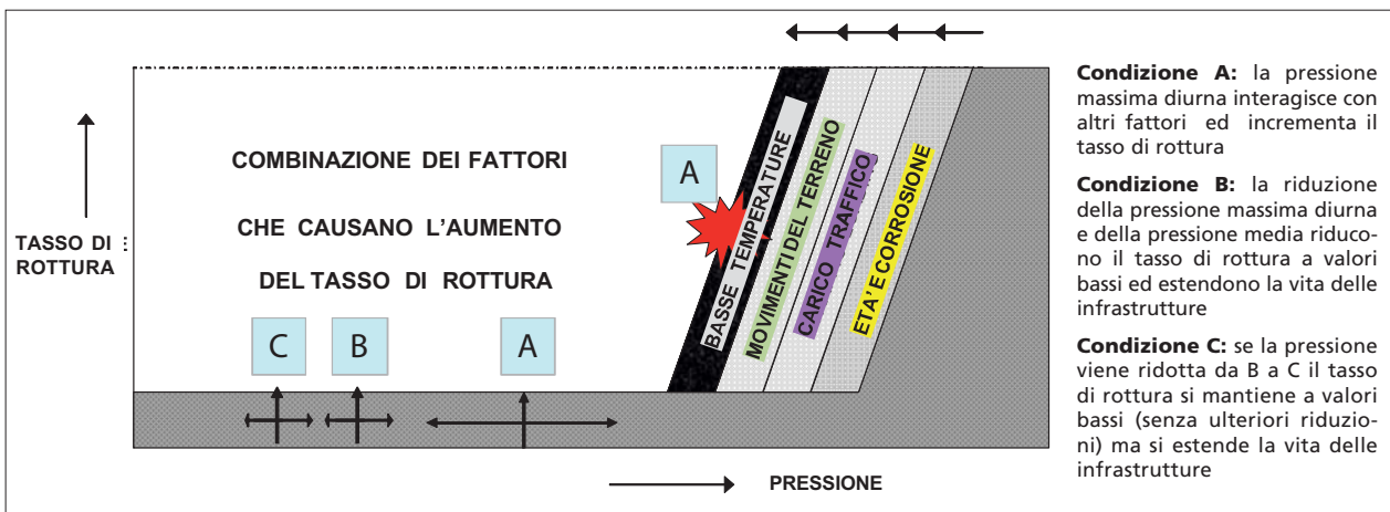
FIGURA 3: INFLUENZA DELLA GESTIONE DELLA PRESSIONE SULLA FREQUENZA DELLE ROTTURE DI RETE E PRESE
