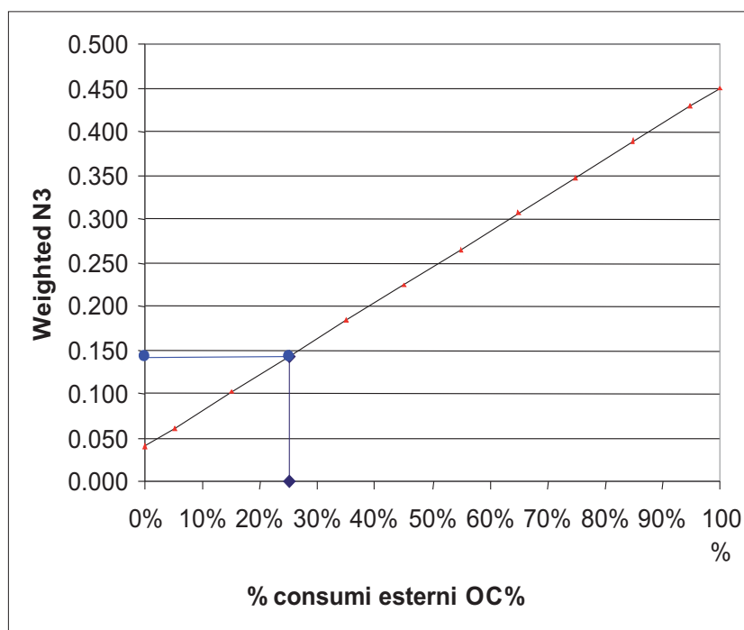
FIGURA 4: SEMPLICE METODO GRAFICO PER LA STIMA DEL VALORE MEDIO PESATO DELL'ESPOLENTE DI CONSUMO N3 (WEIGHTED N3)
