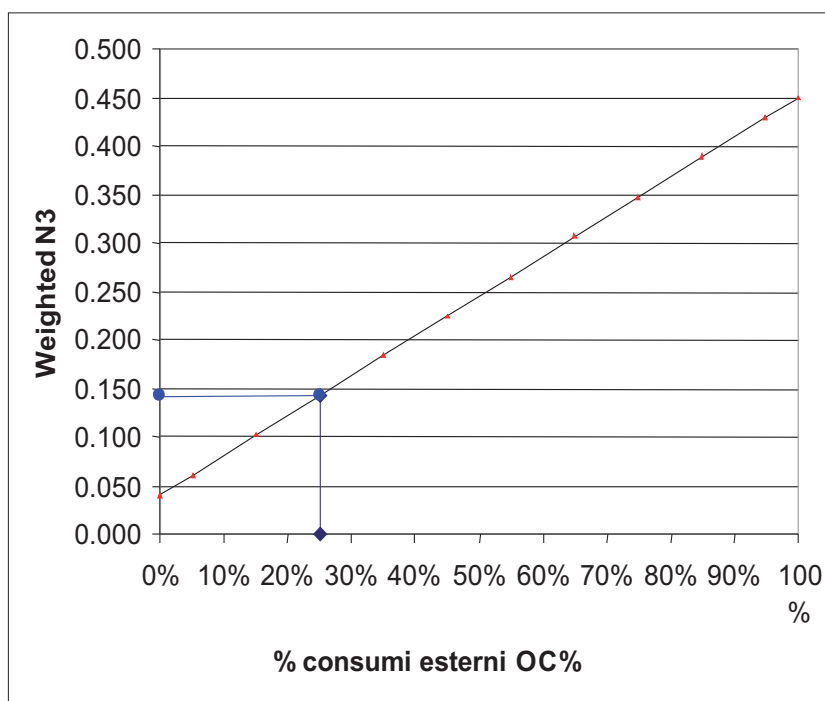
FIGURA 4: SEMPLICE METODO GRAFICO PER LA STIMA DEL VALORE MEDIO PESATO DELL'ESPOSANTE DI CONSUMO N3 (WEIGHTED N3)
